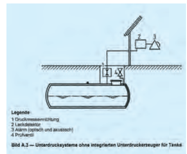
Installation Warnsystem
